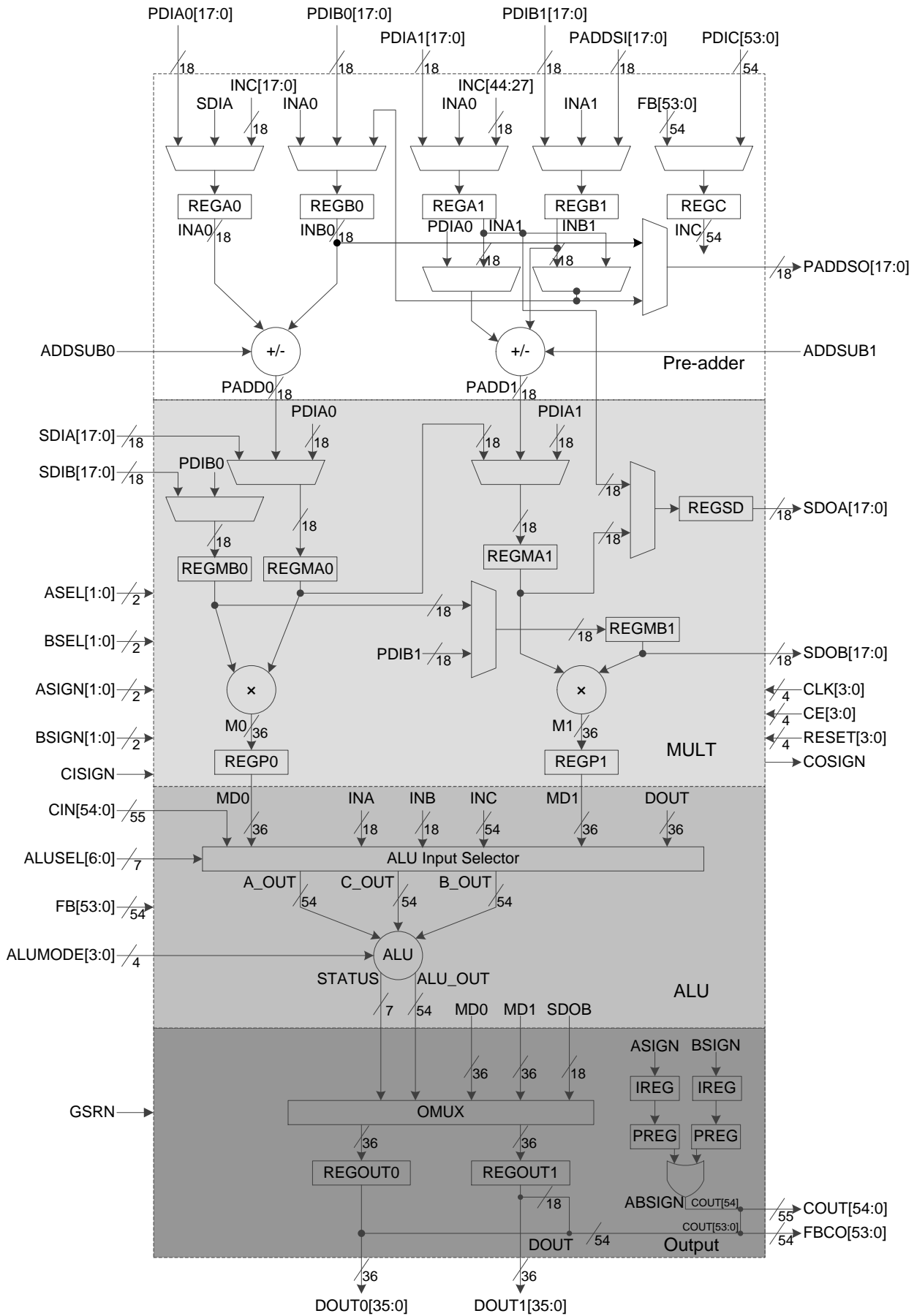
图 3-38 DSP 宏单元
