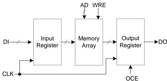
图 3-37 单端口时钟模式
