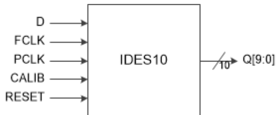
图 3-21 I/O 逻辑的 IDE10 输入示意图
