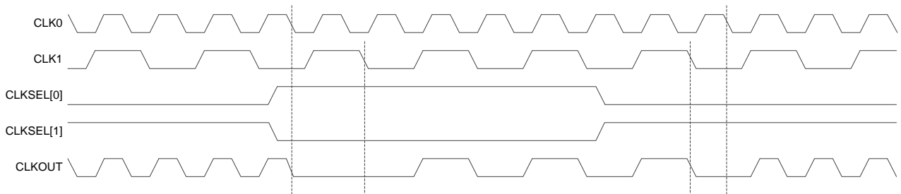
图 3-44 DCS Falling Edge 模式下的时序示意图
