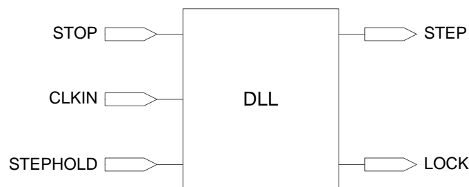
图 3-47 GW2A 的数字锁相环示意图
