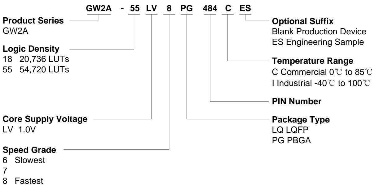
图 5-1 器件命名方法
