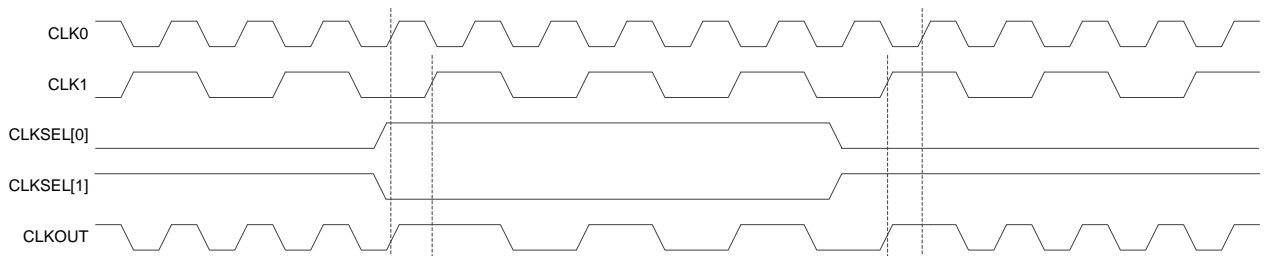
图 3-43 DCS Rising Edge 模式下的时序示意图
