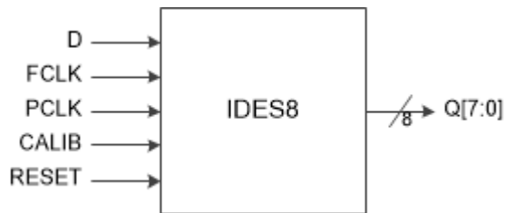
图 3-19 I/O 逻辑的 IDE8 输入示意图
