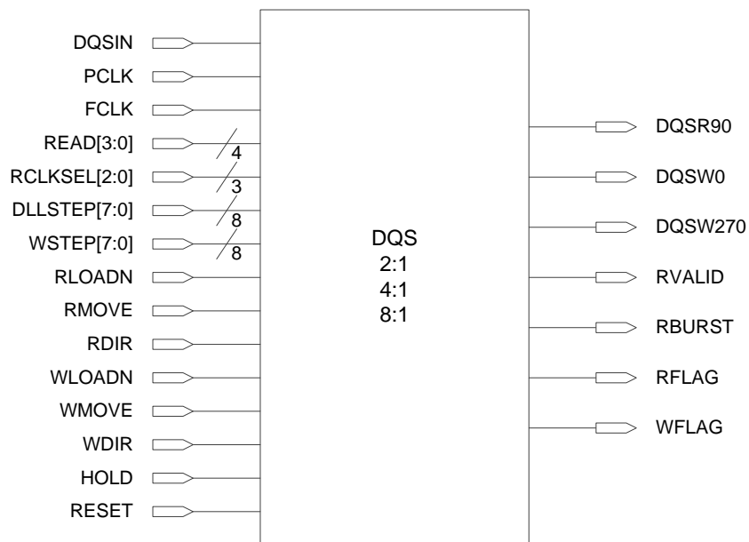
图 3-48 DQS 示意图
