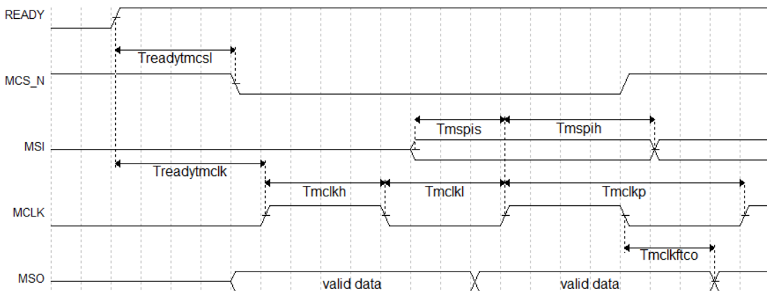
图 4-2 MSPI 编程模式时序示意图
